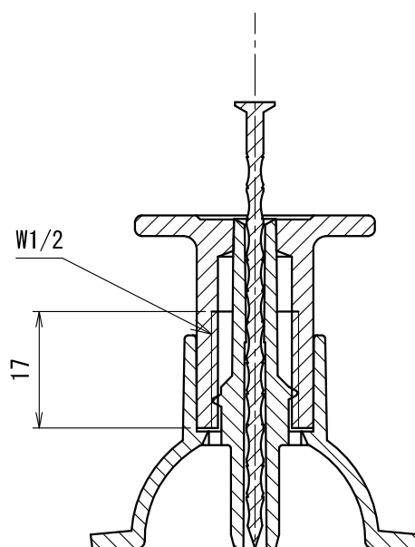
断面 A-A
